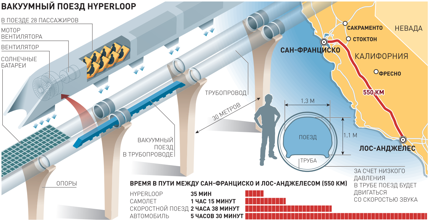
ИДЕЯ ВАКУУМНОГО ПОЕЗДА БЫЛА В 1909 ГОДУ ОПУБЛИКОВАНА ПИОНЕРОМ АМЕРИКАНСКОЙ КОСМОНАУТИКИ РОБЕРТОМ ГОДДАРДОМ. ОН ПРЕДЛОЖИЛ ОРГАНИЗОВАТЬ ДВИЖЕНИЕ АВТОМОБИЛЕЙ В ВАКУУМНОЙ ТРУБЕ НА ОСНОВЕ МАГНИТНОЙ ЛЕВИТАЦИИ СО СКОРОСТЬЮ 1600 КМ/Ч. СОЗДАНИЕМ ВАКУУМНОГО ПОЕЗДА ЗАНИМАЛИСЬ МНОГИЕ ИЗОБРЕТАТЕЛИ, В ЧАСТНОСТИ, В НАЧАЛЕ XX ВЕКА В ТОМСКЕ РУССКИЙ ПРОФЕССОР БОРИС ВЕЙНБЕРГ, А В 30-е ГОДЫ НЕМЕЦКИЙ ИНЖЕНЕР ГЕРМАН КЕМПЕР, НО ВСЕ ЭТИ ПРОЕКТЫ ТАКИ НЕ БЫЛИ РЕАЛИЗОВАНЫ. ПОМЕШАЛИ ВОЙНЫ, НО ГЛАВНОЕ, ЧТО МНОГИЕ ТЕХНОЛОГИИ ЕЩЕ НЕ БЫЛИ ГОТОВЫ К ТАКИМ ПРORYВНЫМ ПРОЕКТАМ. СЕЙЧАС МОЖНО СКАЗАТЬ, ЧТО ИХ ВРЕМЯ ПРИШЛО. И ЭТО НЕ ТОЛЬКО ПРОЕКТ МАСКА. НАПРИМЕР, КИТАЙ НАМЕРЕН К 2020 ГОДУ В ПОДЗЕМНОМ ТУННЕЛЕ ПУСТИТЬ ВАКУУМНЫЙ ПОЕЗД СО СКОРОСТЬЮ ОКОЛО 1000 КМ/Ч. ПЛАНЫ СТРОИТЕЛЬСТВА ПОДОВОДНОГО ТРАНСАТЛАНТИЧЕСКОГО ТУННЕЛЯ ДЛЯ СВЕРХЗВУКОВЫХ ПОЕЗДОВ НА МАГНИТНОЙ ПОДУШКЕ ПРЕДЛАГАЕТ ОДИН ИЗ ПРОЕКТИРОВЩИКОВ ЕВРОПЕЙСКОЙ АМЕРИКАНСКОЙ КОМПАНИИ ФРЭНК ДЭВИДСОН. ФИНСКИЕ ИНЖЕНЕРЫ РАЗРАБОТАЛИ ПРОЕКТ ПОДОВОДНОГО ТУННЕЛЯ МЕЖДУ ХЕЛЬСИНКИ И ТАЛЛИНОМ, ГДЕ БУДЕТ КУРСИРОВАТЬ ВАКУУМНЫЙ ПОЕЗД СО СКОРОСТЬЮ 1600 КИЛОМЕТРОВ В ЧАС.
